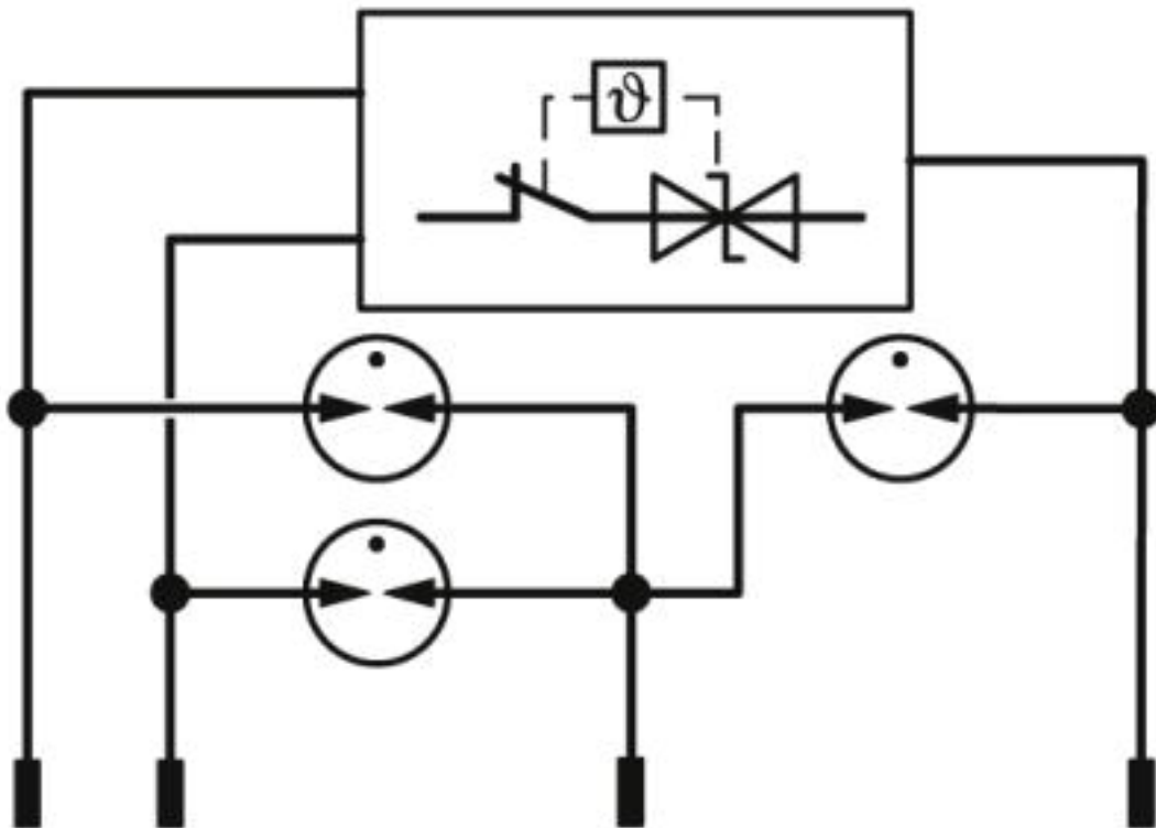
电路图
